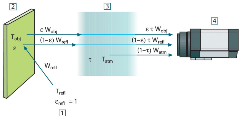
그림 43.1 일반 열 측정 상황의 개략적 재현. 1: 주변 환경; 2: 물체; 3: 대기; 4: 카메라
