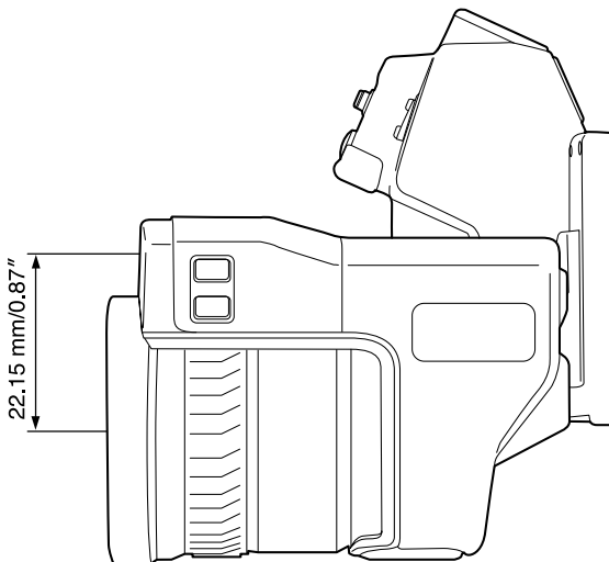
그림 12.1 이 그림은 레이저 포인터와 적외선 렌즈 중심 간의 위치 차이를 보여줍니다.
