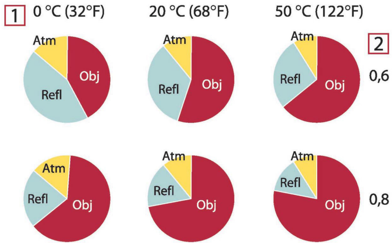
그림 43.3 다양한 측정 조건 하에서 방사원의 상대적 중요도(LW 카메라). 1: 물체 온도; 2: 방출량; Obj: 물체 방사; Refl: 반사된 방사; Atm: 대기 방사. 고정 매개변수: \tau = 0.88 ; T_{refl} = 20^{\circ}\text{C} ; T_{atm} = 20^{\circ}\text{C} .
