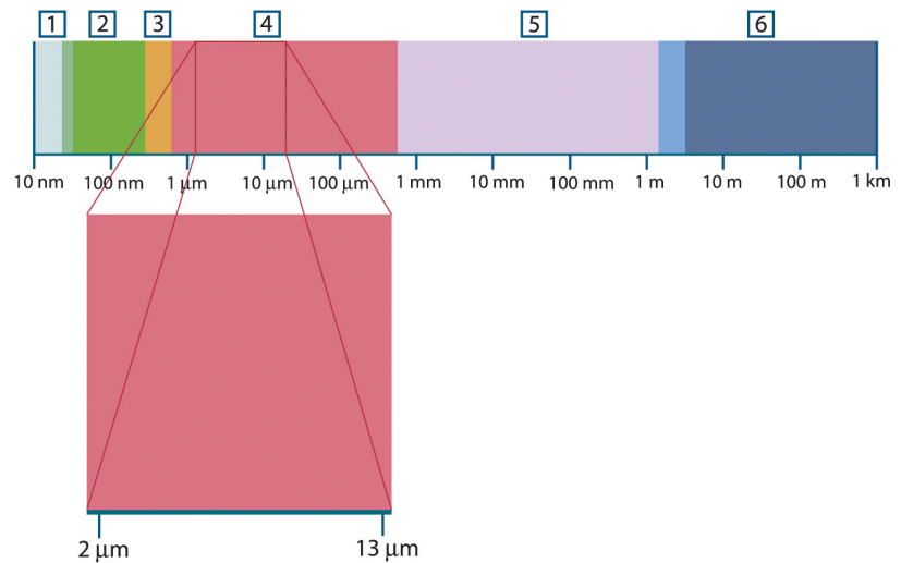
그림 42.1 전자기 스펙트럼 1: X-레이; 2: 자외선; 3: 가시선; 4: 적외선; 5: 극초단파; 6: 무선파
