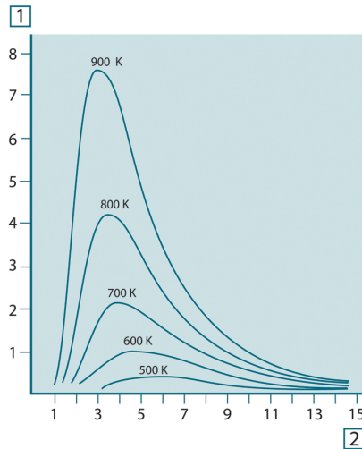
그림 42.4 플랑크 복사 공식에 따르면 흑체 분광 복사 에너지 방출량은 다양한 절대 온도에 따라 점으로 표시됩니다. 1: 분광 방출 스펙트럼( \text{W/cm}^2 \times 10^3(\mu\text{m}) ); 2: 파장( \mu\text{m} )
