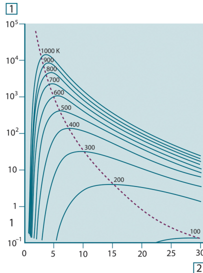
그림 42.6 플랑크 곡선은 모든 종이 간격으로 100 K에서 1000 K까지 점으로 곡선을 그립니다. 점선은 Wien의 법칙에 의해 설명된 것처럼 각 온도에 최대 복사 에너지 방출량의 궤적을 나타냅니다. 1: 분광 복사 에너지 방출량( \text{W}/\text{cm}^2 (\mu\text{m}) ); 2: 파장( \mu\text{m} )
