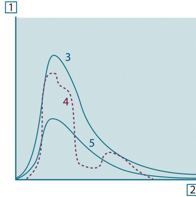
그림 42.8 세 가지 유형의 방사기의 분광 복사 방출량. 1: 분광 복사 방출량; 2: 파장; 3: 흑체; 4: 선택적 방사기; 5: 회색체
