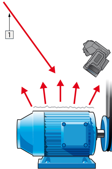
그림 39.5 알루미늄 호일의 추정 온도 측정
