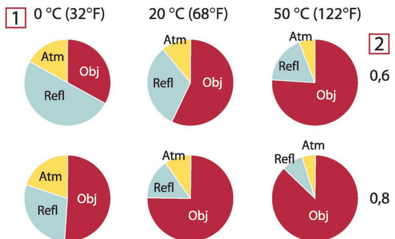
그림 43.2 다양한 측정 조건 하에서 방사원의 상대적 중요도(SW 카메라). 1: 물체 온도; 2: 방출량; Obj: 물체 방사; Refl: 반사된 방사; Atm: 대기 방사. 고정 매개변수: \tau = 0.88 ; T_{refl} = 20^{\circ}\text{C} ; T_{atm} = 20^{\circ}\text{C} .
