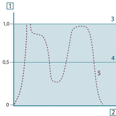
그림 42.9 세 가지 유형의 방사기의 분광 복사 방출량. 1: 분광 복사 방출량; 2: 파장; 3: 흑체; 4: 회색체; 5: 선택적 방사기
