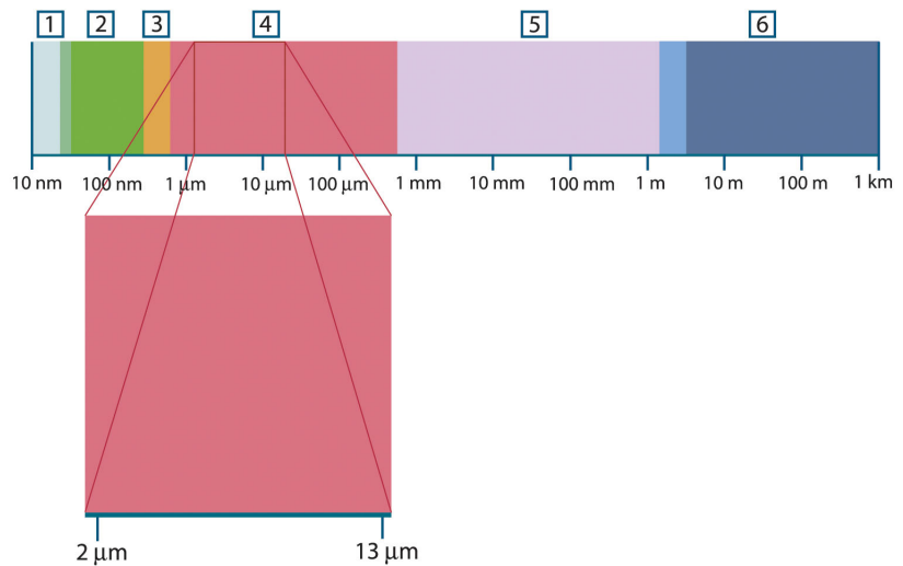
그림 36.1 전자기 스펙트럼 1: X-레이; 2: 자외선; 3: 가시선; 4: 적외선; 5: 극초단파; 6: 무선파
