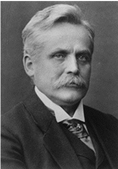
그림 36.5 Wilhelm Wien(1864–1928)
