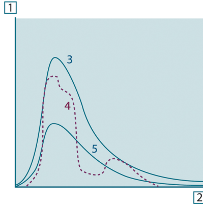
그림 36.8 세 가지 유형의 방사기의 분광 복사 방출량. 1: 분광 복사 방출량; 2: 파장; 3: 흑체; 4: 선택적 방사기; 5: 회색체
