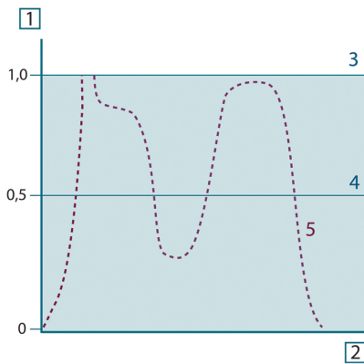
그림 36.9 세 가지 유형의 방사기의 분광 복사 방출량. 1: 분광 복사 방출량; 2: 파장; 3: 흑체; 4: 회색체; 5: 선택적 방사기
