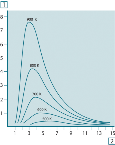
그림 36.4 플랑크 복사 공식에 따르면 흑체 분광 복사 에너지 방출량은 다양한 절대 온도에 따라 점으로 표시됩니다. 1: 분광 방출 스펙트럼(W/cm 2 × 10 3 (μm)); 2: 파장(μm)
